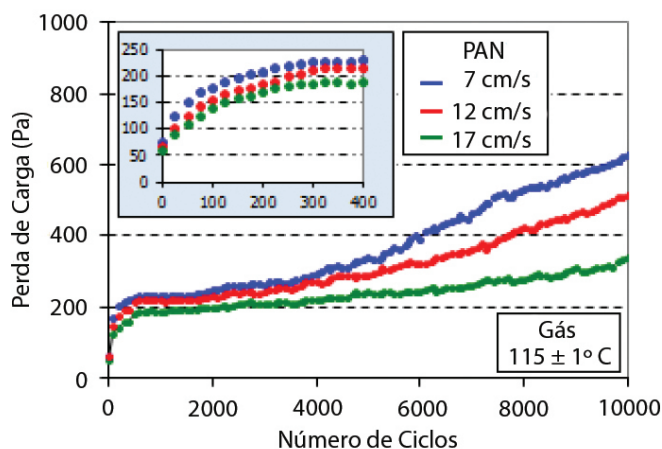
Figura 6: Perda de carga - PAN a quente
