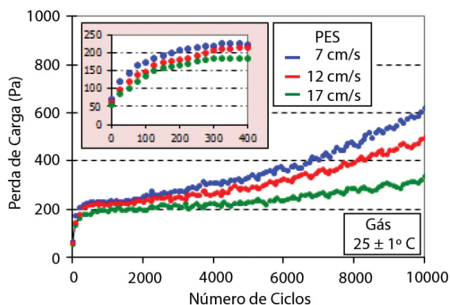
Figura 7: Perda de carga - PES a frio
