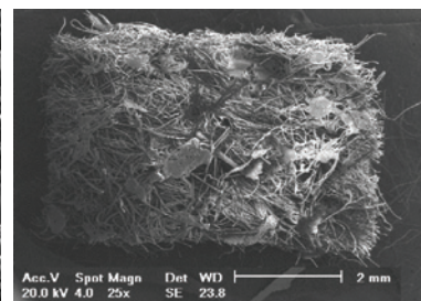
Figura 14: Micrografia de PI a 240°C
