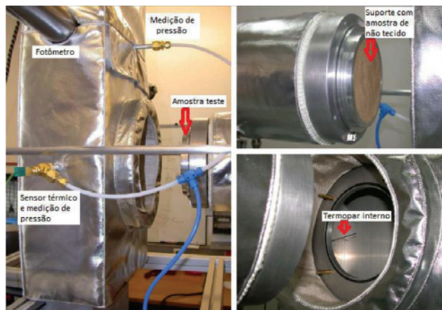
Figura 3 - Parte interna do duto aberto com a amostra de não tecido
