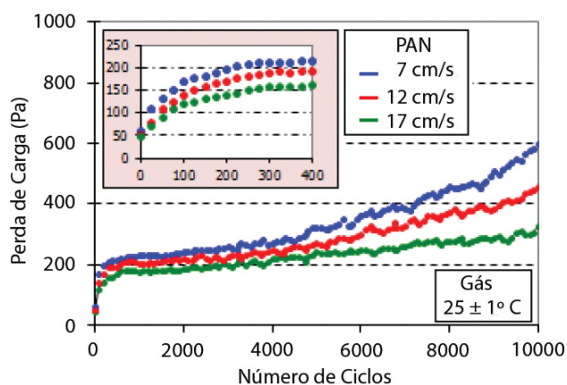
Figura 5: Perda de carga - PAN a frio
