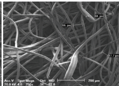
Figura 12: Micrografia de PAN
