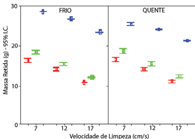
Figura 15 - Limites de confiança de 95% para massa retida pela ANOVA
