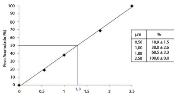
Figura 4 - Distribuição granulométrica do particulado de PEBD
