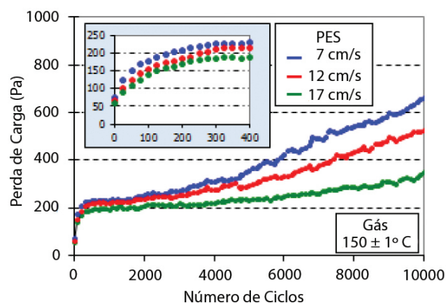
Figura 8: Perda de carga - PES a quente
