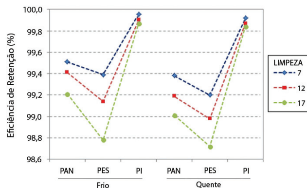
Figura 16 - Eficiência a frio e a quente
