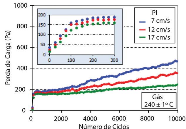
Figura 10: Perda de carga - PI a quente
