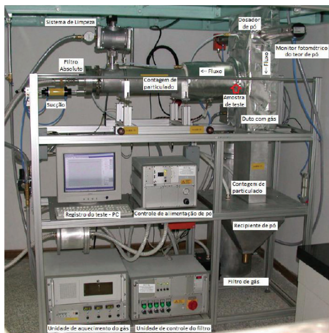
Figura 2 - Partes identificadas do simulador de filtração
