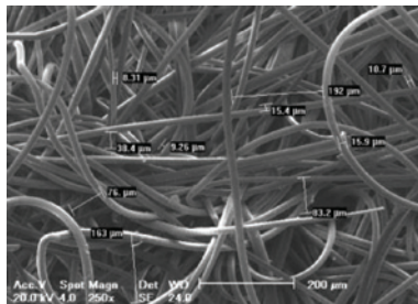
Figura 11: Micrografia de PES
