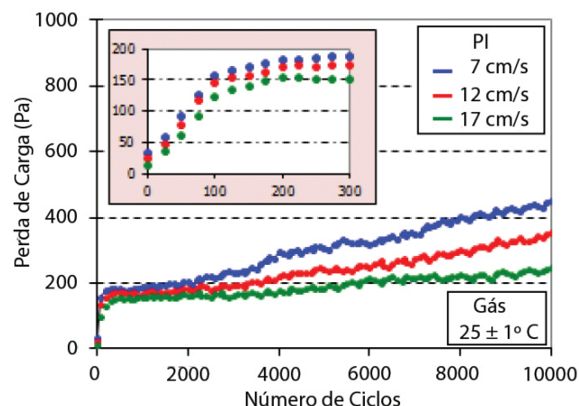
Figura 9: Perda de carga - PI a frio
